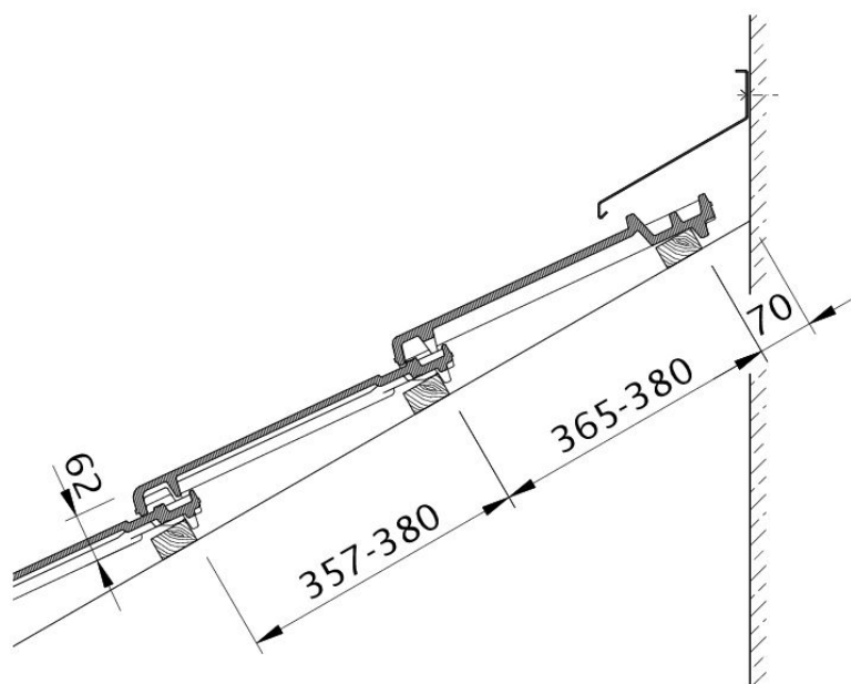
Tehnički crtež proizvoda RATIO WMF WMF
