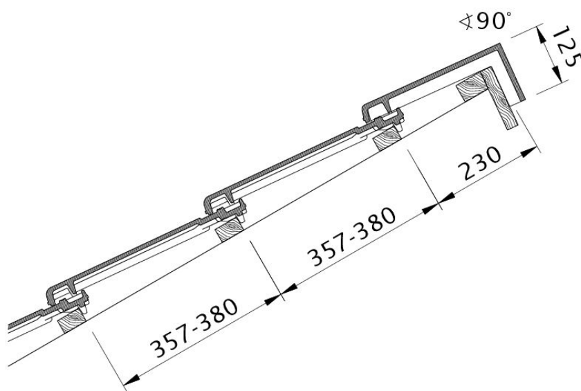
Tehnički crtež proizvoda RATIO PDA PDA
