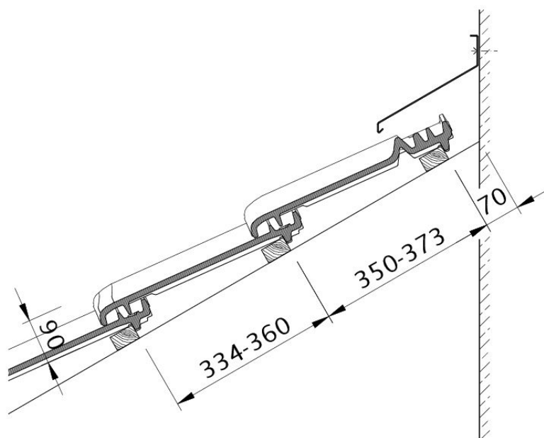
Tehnički crtež proizvoda MZ3 WMF WMF
