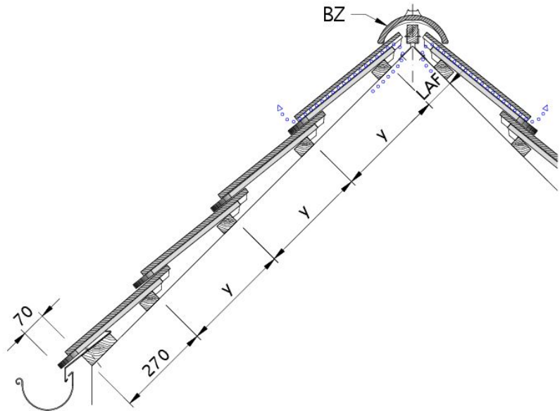
Tehnički crtež proizvoda KLASSIK DQF DQK-2
