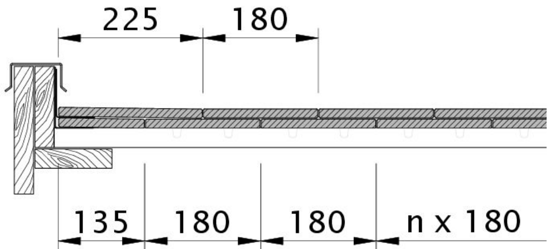
Tehnički crtež proizvoda KLASSIK OBR OBR
