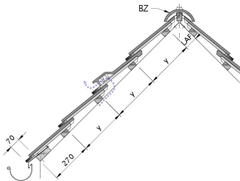
Tehnički crtež proizvoda KLASSIK DQF DQK-1
