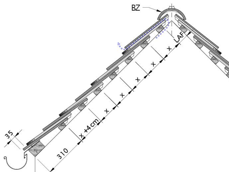
Tehnički crtež proizvoda KLASSIK DQF DQD-3
