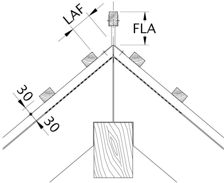
Tehnički crtež proizvoda KLASSIK LAF LAF
